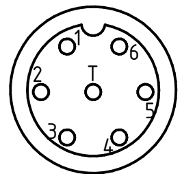
Schema elettrico - Wiring diagram Diagrama de cableado
